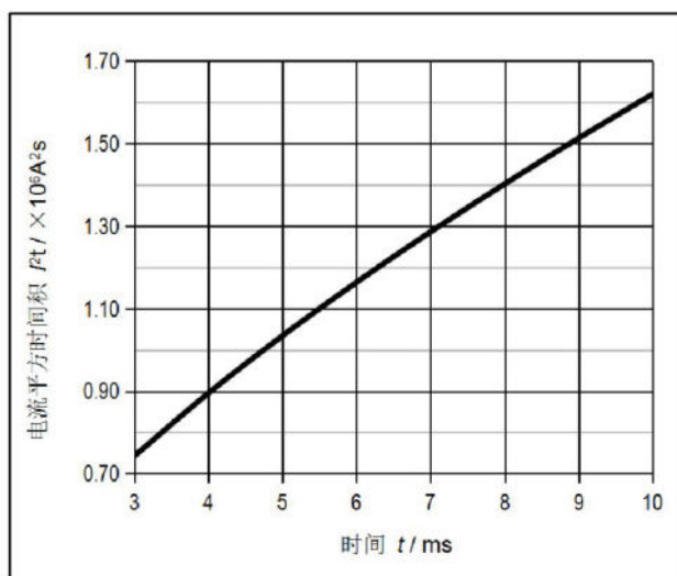
图5. I^2t 特性曲线
