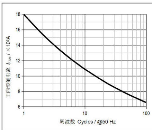
图4. 浪涌电流与周波数的关系曲线
